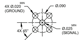
MDCX および MDHC PCB フットプリント
